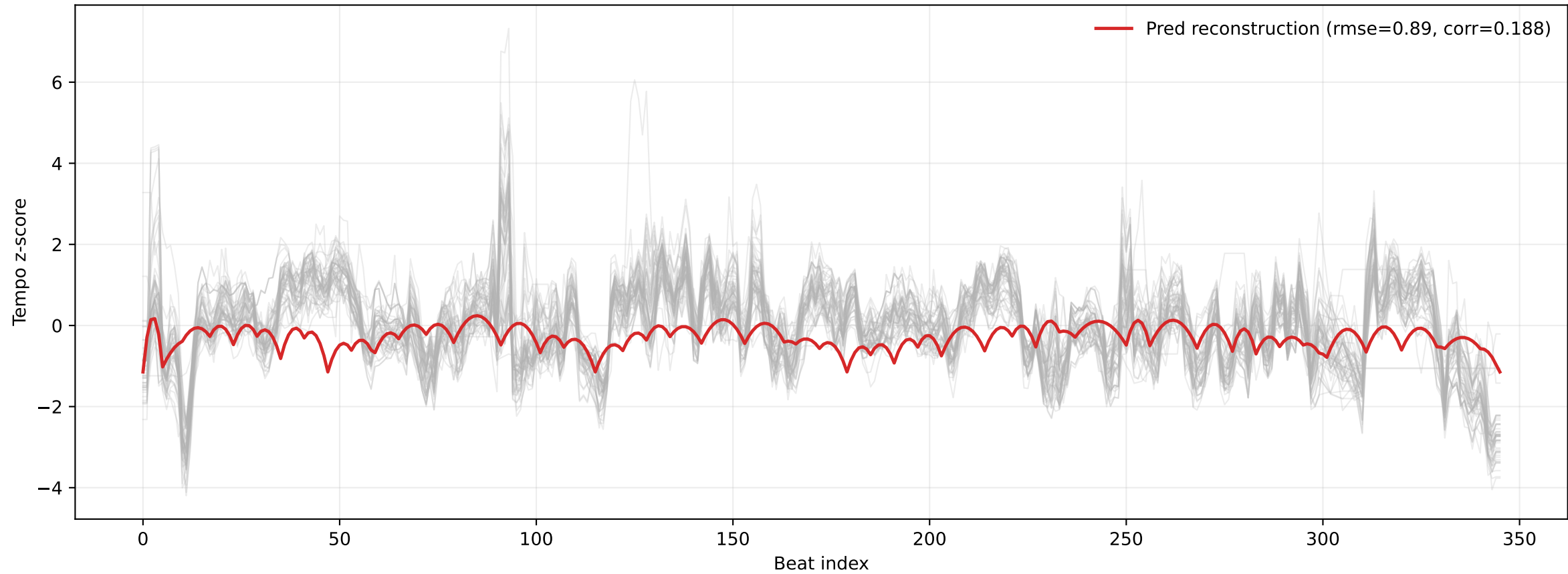
ludwig_van_beethoven_piano_sonata_no_31_in_a_flat_major_op_110_i_moderato_cantabile_molto_espressivo: Pred reconstruction vs ALL performer tempo curves
